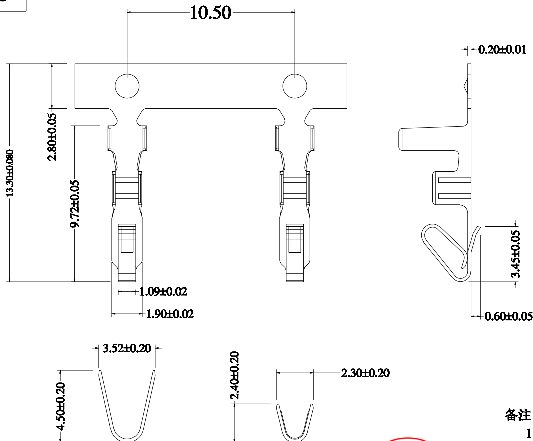
电镀后收料示意图 顺收线夹向上
