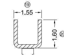
SECTION: C-C SCALE: 1:1
