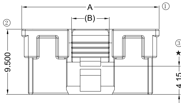
03~15P Shape
